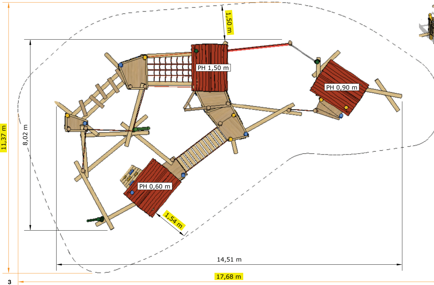
Aufsicht/ Sicherheitsbereich
