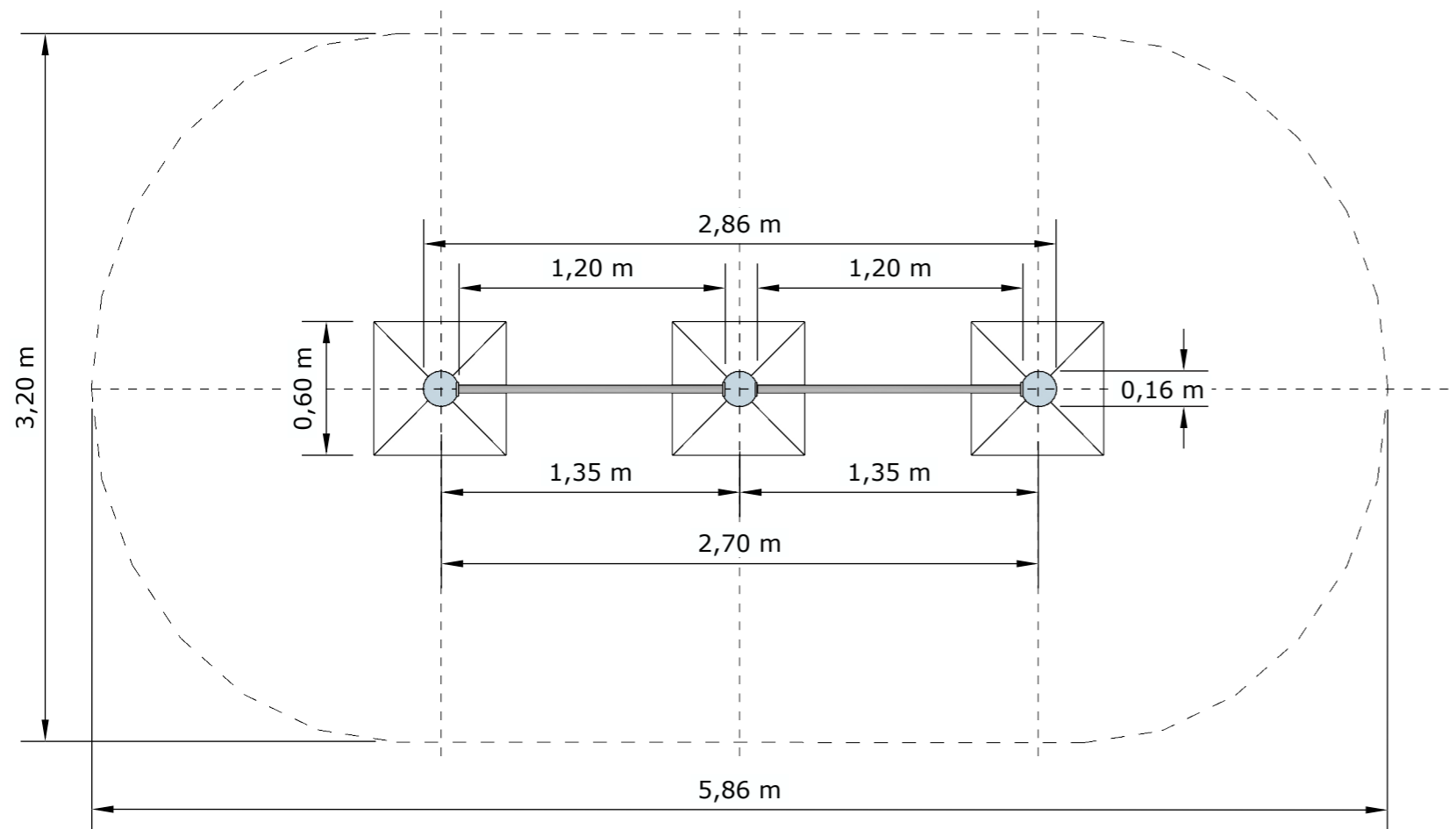
Aufsicht/ Fundament – Maßstab 1:30
