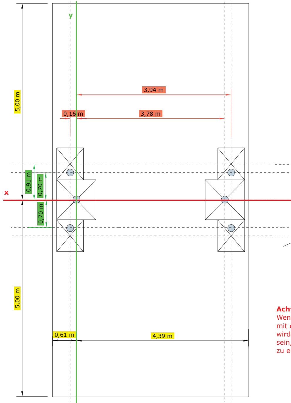
Fundamentplan xy – Maßstab 1:40
