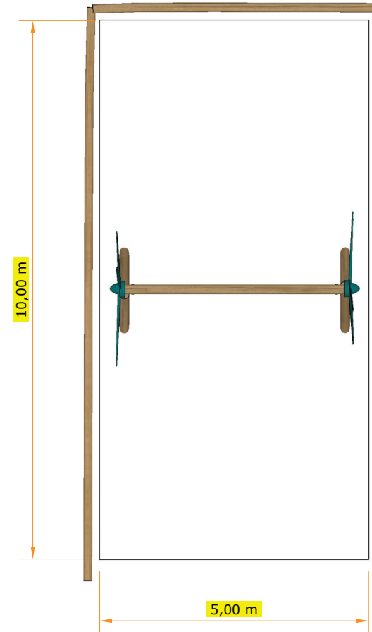
Sicherheitsbereich – Maßstab 1:70
