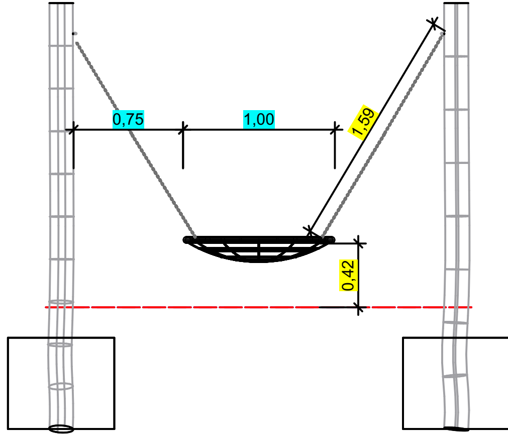
Fundamentdarstellung Seitenansicht:
