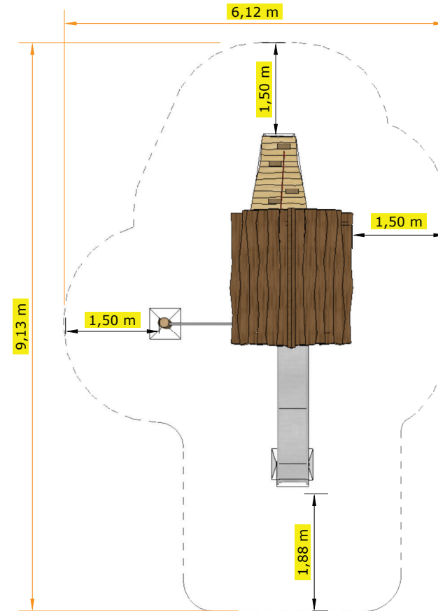
Sicherheitsbereich – Maßstab 1:60
