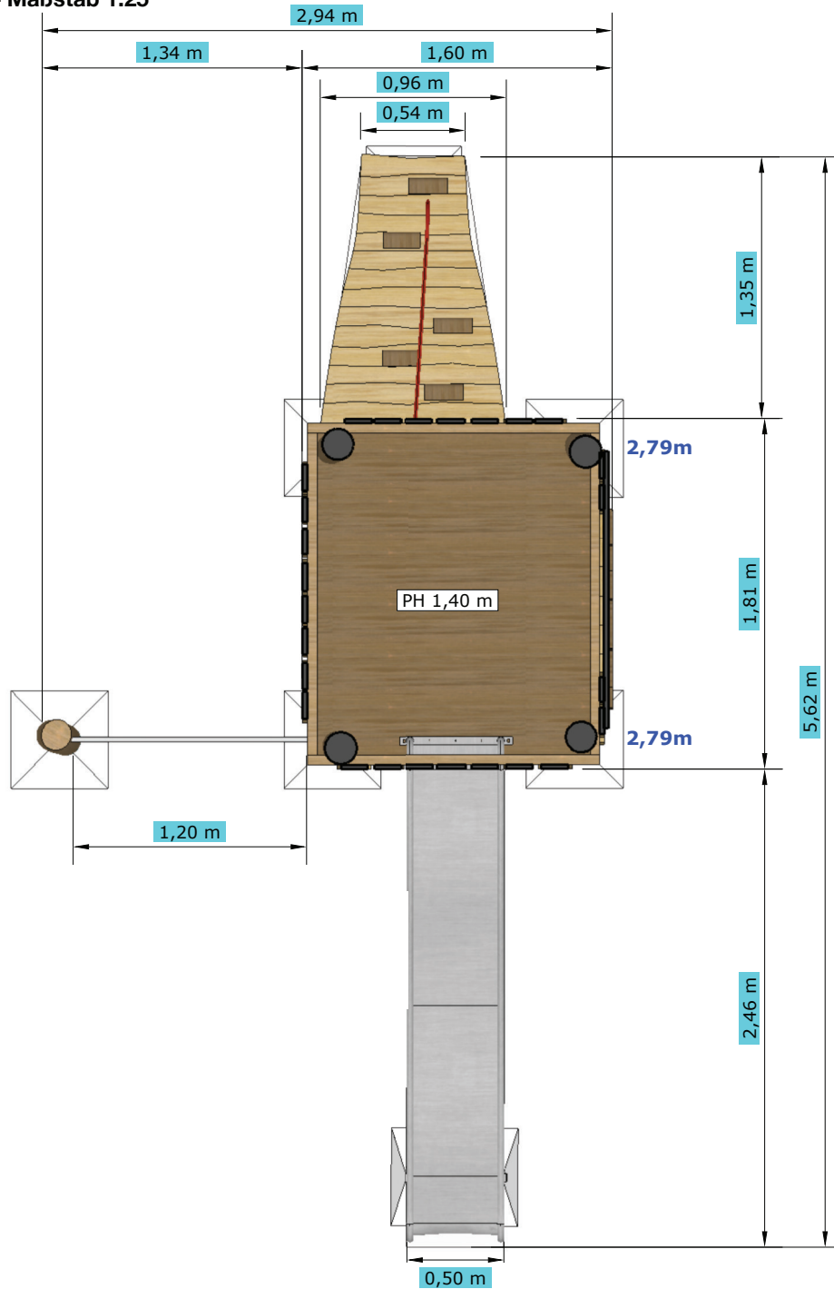
Schnitt – Maßstab 1:25
